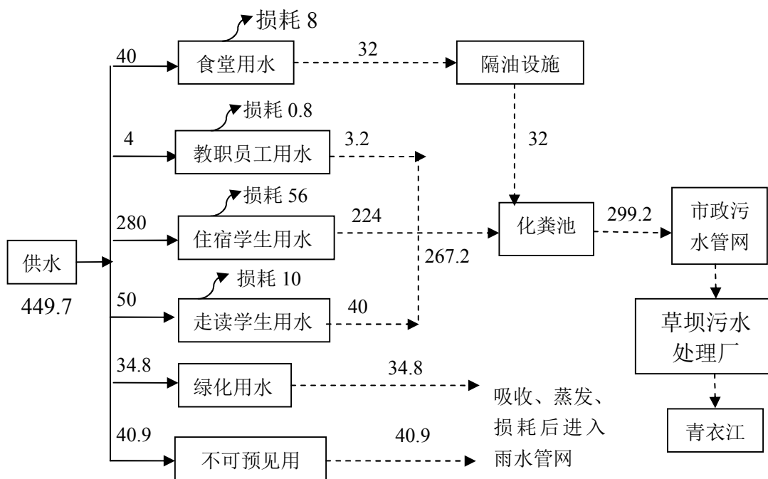
图 5-2 项目水平衡图 (单位: m 3 /d)
